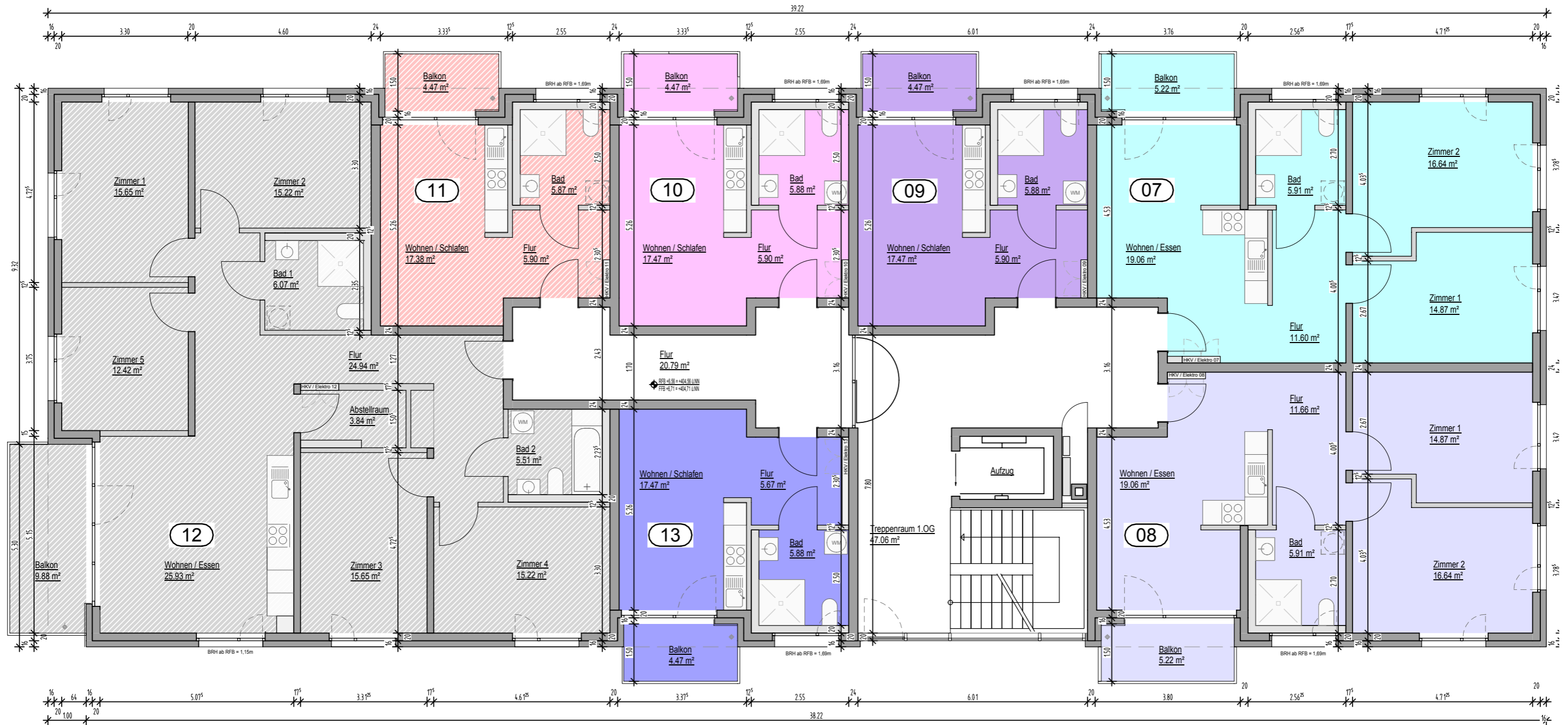
Grundriss 2. Obergeschoss
